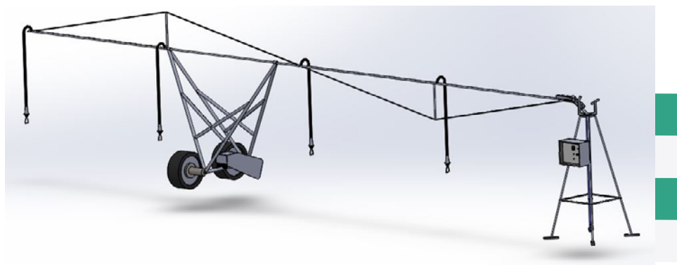
Figura 1: Projeto do pivô central feito em programa de desenho assistido por computador.
